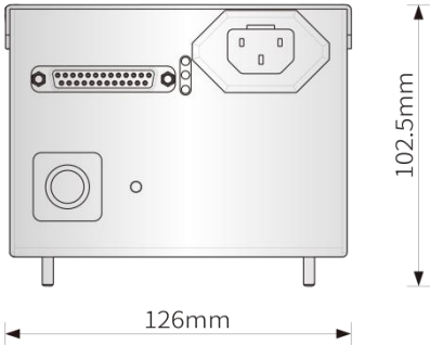
主视图
