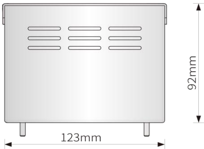
后视图
